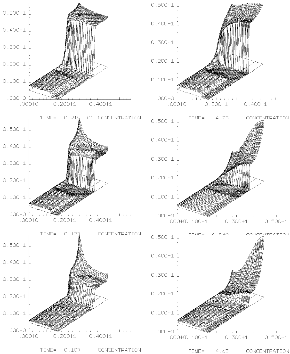
Рис. 4.6.7. Распределение примеси. Скорость роста: 0.0001 см/сек - верхний ряд, 0.0005 см/сек - средний ряд, 0.001 см/сек - нижний ряд; ускорение силы тяжести: наземное g_0 - левый столбец, орбитальное 0.001g_0 - правый столбец. Результат получен с помощью программы АСТРА
