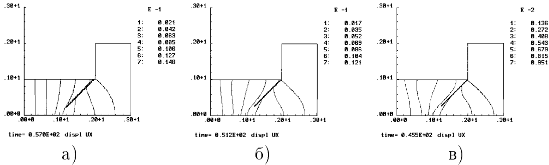
Рис. 4.4.5. Зависимость решения для упругопластического материала от шага пространственной сетки.
