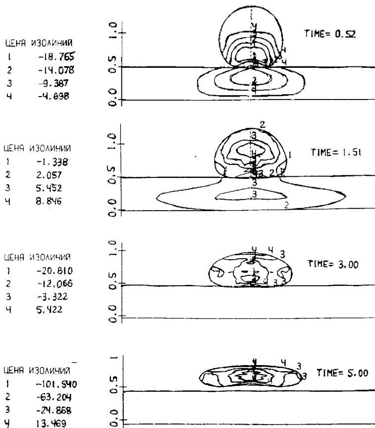
Рис. 4.3.2. Удар алюминиевым шаром в стальную преграду.
