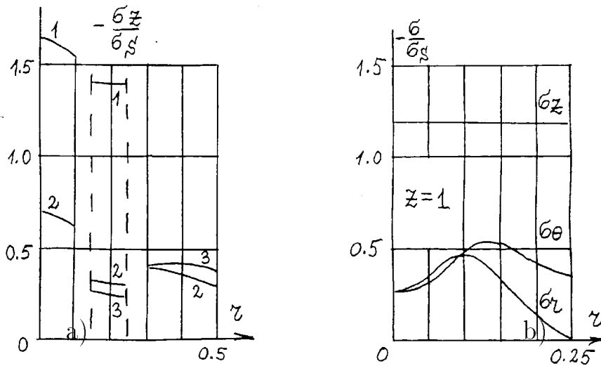
Рис. 4.2.2. Сжатие гребенчатого соединения двух разнородных упругопластических тел вращения а) - распределение контактных напряжений в зубах ( сечения z = 0.9 , z = 0.55 , z = 0.2 ); б) - распределение напряжений в сечении z = 1
