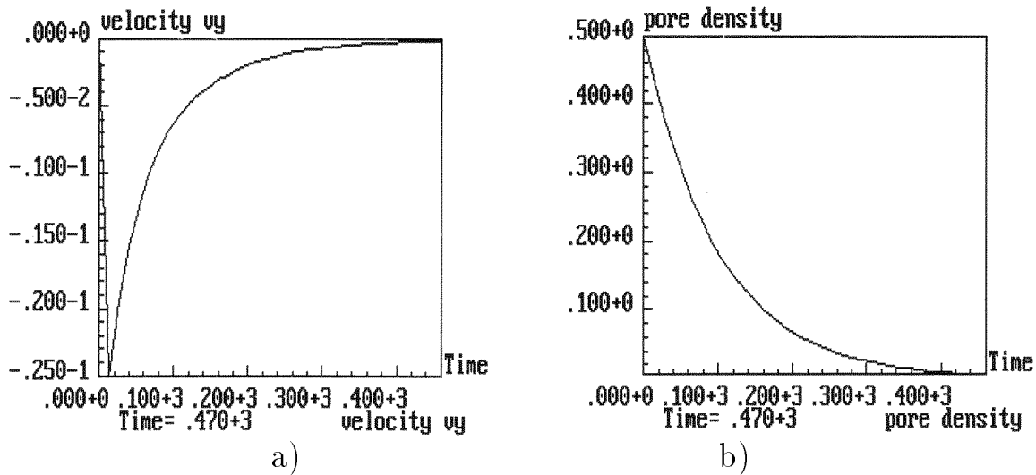
Рис. 4.5.3. Спекание (однородный процесс). Рассчитанные истории граничной скорости (a) и пористости (b).
