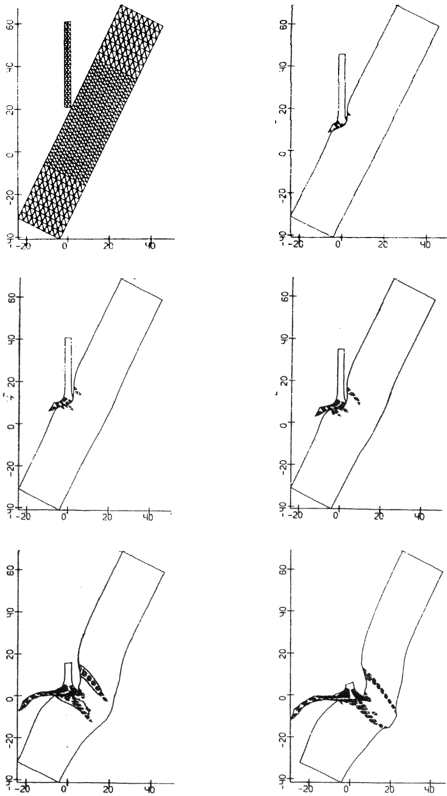
Рис. 4.4.10. Соударение пластин под углом с учетом разрушения. Эволюция зон разрушения. Окончательно пластина раскололась на три части. Ударник разрушен полностью.
