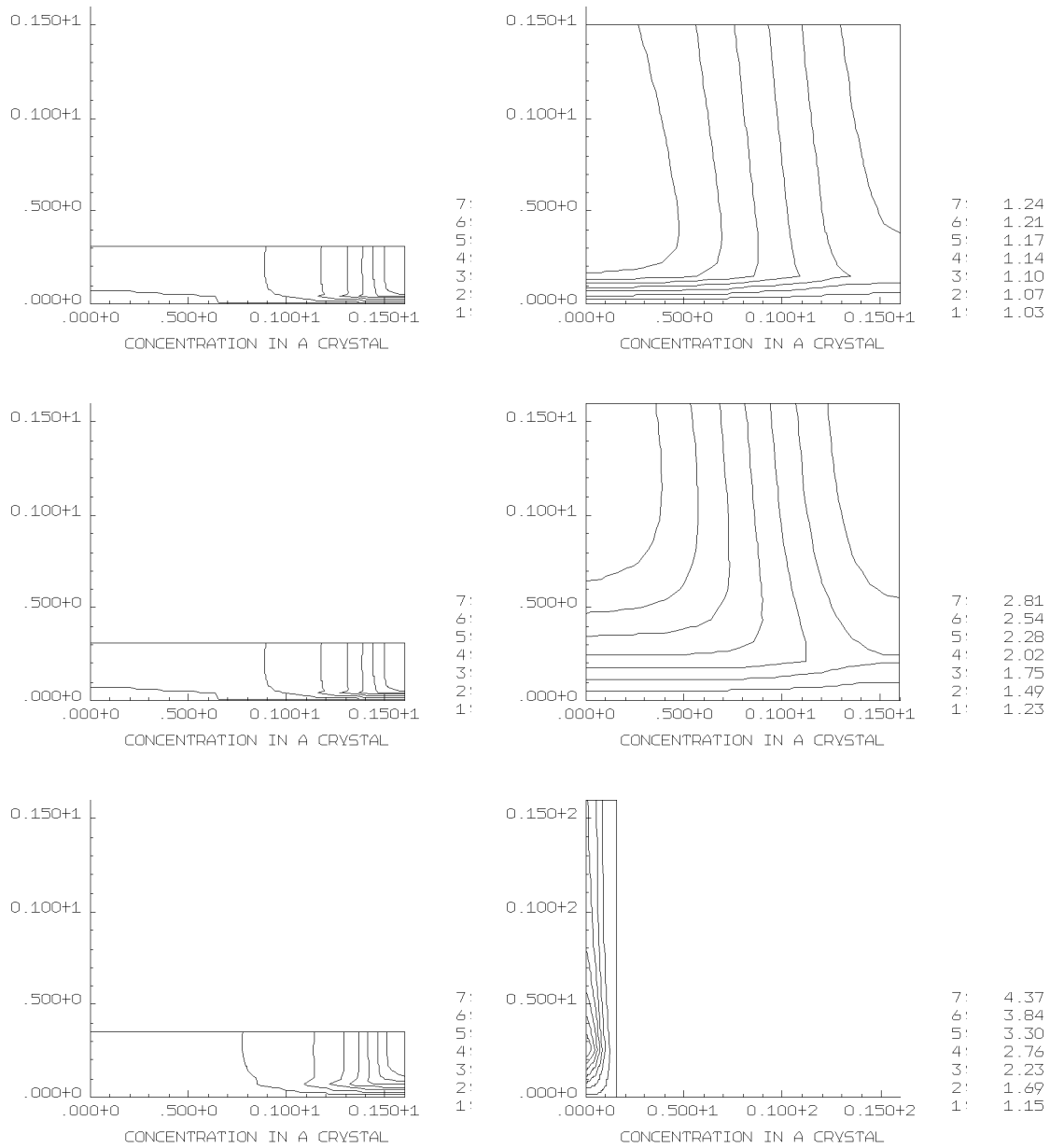
Рис. 4.6.8. Распределение концентрации Ga в кристалле Ge для 6 случаев процесса роста кристалла из работы Острогорского. Левая колонка (сверху вниз): g = g_0 , V_s = 0.0001 \text{ cm/sec}, 0.0005 \text{ cm/sec}, 0.001 \text{ cm/sec} ; правая колонка: g = 0.001g_0 . Результат получен с помощью программы АСТРА.
