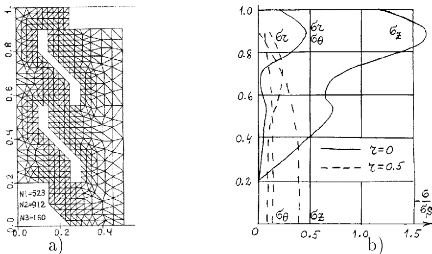
Рис. 4.2.1. Сжатие гребенчатого соединения двух разнородных упругопластических тел вращения а) расчетная сетка; б) распределение напряжений вдоль оси z на внешней поверхности ( r = 0,5 ).
