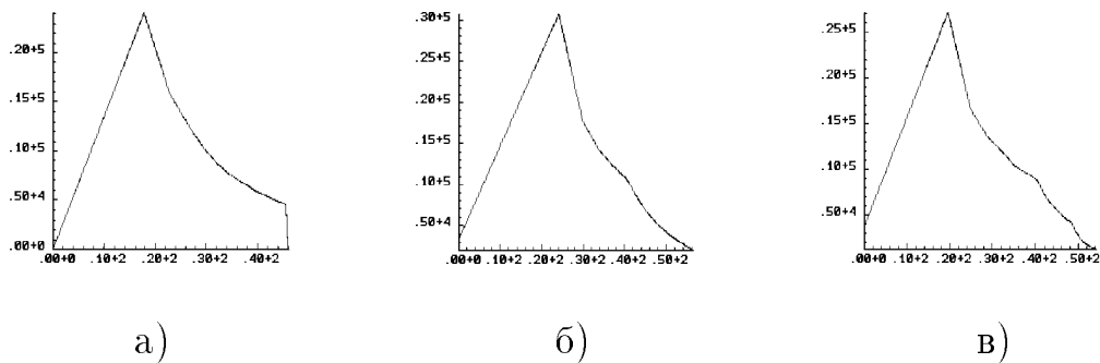
Рис. 4.4.4. Изменение безразмерного шага по времени, отнесенного к величине шага Куранта для явных схем и выбираемого из условий точности, от величин 10^4 для квазистатики в начале процесса до величин порядка 1 при распространении зон разрушения.
