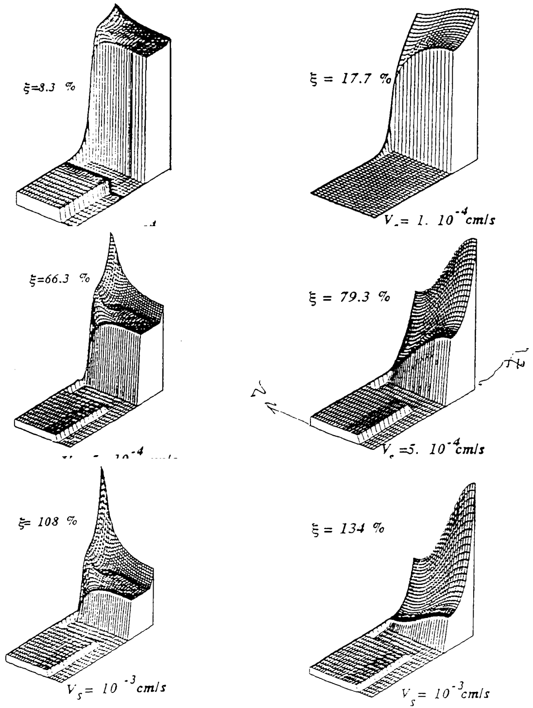
Рис. 4.6.6. Распределение примеси в расплаве в методе погруженного нагревателя (результат А. Острогорского).
