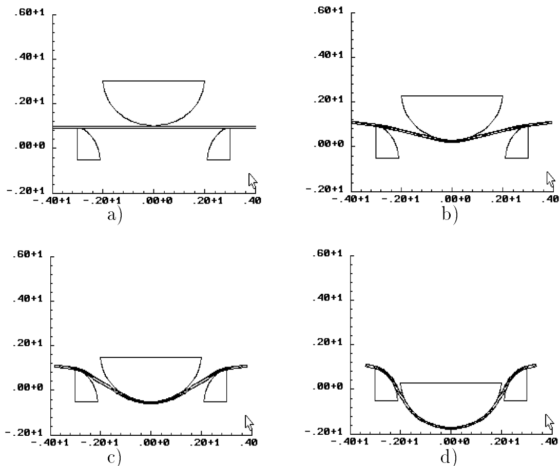
Рис. 4.2.4. Формование упругопластической алюминиевой чашки
