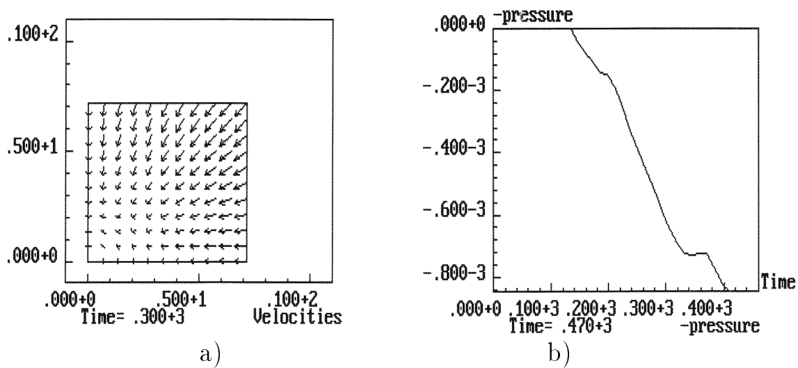
Рис. 4.5.3. Спекание (однородный процесс). Рассчитанные поле скоростей (a) и история давления (b), которое практически равно нулю, как и должно быть.
