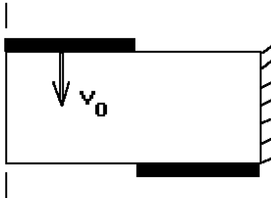
Рис. 4.4.6. Процесс резки металлического листа. Расчетная схема.
