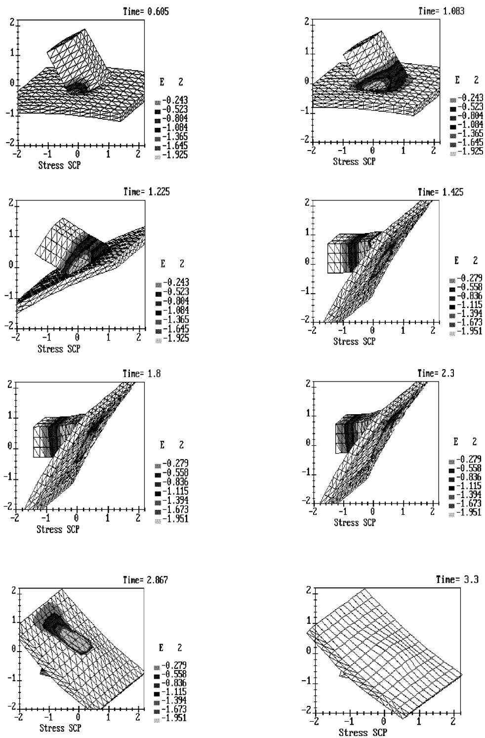
Рис. 4.3.5. Удар двух тел под углом.
