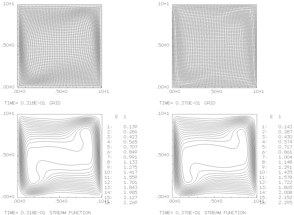
Рис. 4.7.3. Поведение адаптивной сетки, управляемой уравнениями нелинейной термоупругости, и функции тока в задаче о термогравитационной конвекции вязкой несжимаемой жидкости при числе Грасгофа Gr =_{10} 7 для двух случаев выбора адаптационной функции: функция тока (левая колонка) и завихренность (правая колонка). Результат получен с помощью программы АСТРА.
