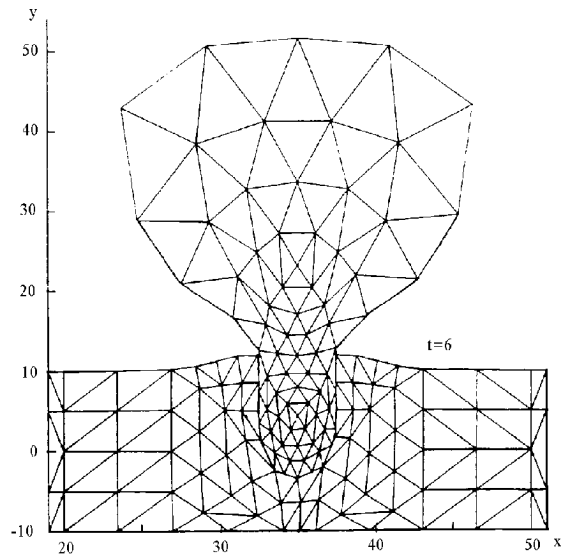
Рис. 4.3.7. Исходная расчетная сетка. Показана часть области решения в окрестности заряда. Мелкая квазиравномерная сетка покрывает заряд. Более крупные ячейки покрывают область грунта. Между грунтом и зарядом вначале имеется небольшой зазор.
