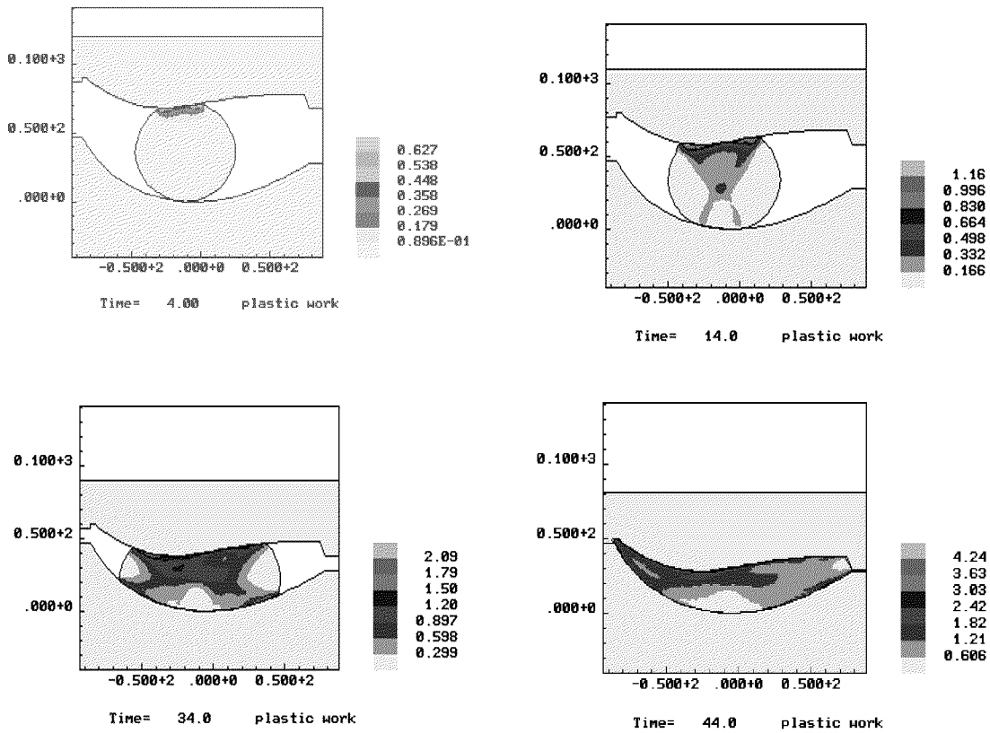
Рис. 4.2.5. Формование лопатки турбины.
