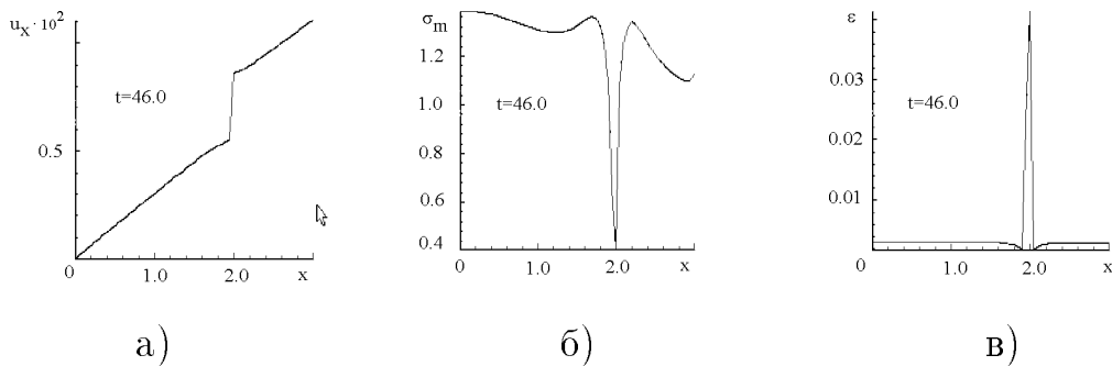
Рис. 4.4.3. Графики горизонтального смещения (а), среднего напряжения (б) и максимальной деформации (в) вдоль горизонтальной линии y = 0.6 для случая разрушения упругого материала, показанного на Рис. 4.8.1.2а. В остальных случаях качественное поведение такое же.
