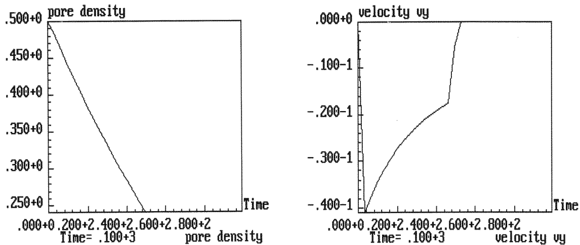
Рис. 4.5.2. Холодное прессование. Результаты проверочного расчета соответствуют аналитическому решению и представлениям о физике процесса.
