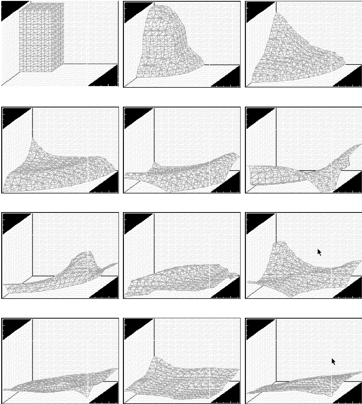
Рис. 4.6.11. Обрушение водяной колонны в замкнутом бассейне. Результат получен с помощью программы АСТРА.
