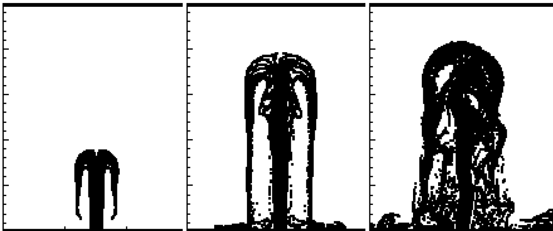
Рис. 4.6.13. Фонтан и лужа от вертикальной струи. Результат получен с помощью программы АСТРА.
