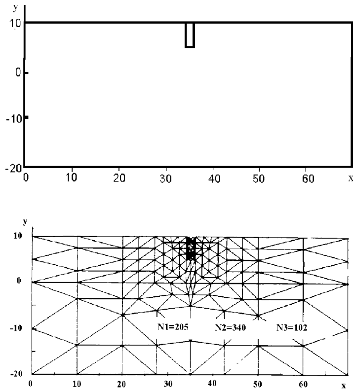
Рис. 4.3.6. Образование воронки при взрыве. а - конфигурация деформируемых тел ( t=0 ) ; б - расчетная сетка;
