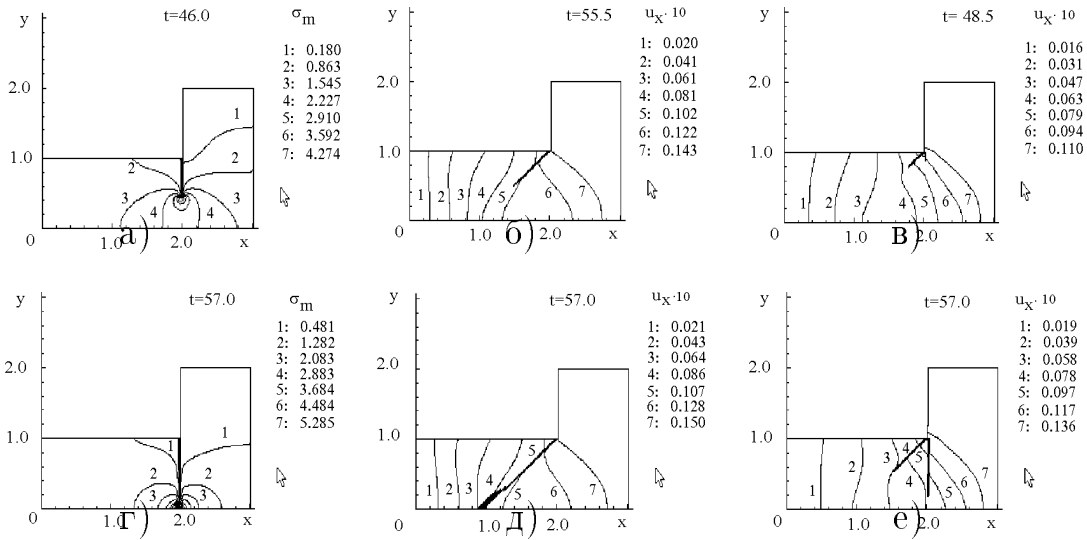
Рис. 4.4.2. Моды процесса разрушения, изолинии среднего напряжения \sigma_m и горизонтального перемещения u_x для случаев упругого материала (а,г), упругопластического материала (б,д), упругопластического материала при совместном действии растяжения и нагрева узкой вертикальной зоны под концентратором (в,е). Показаны средняя (а,б,в) и финальная (г,д,е) стадии процесса.
