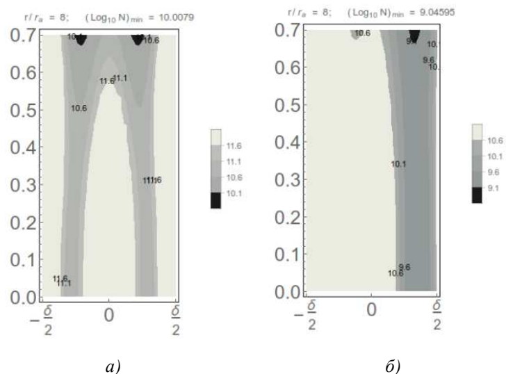
Рис. 1. Изолинии логарифма долговечности в прямоугольном сечении на внешнем ободе диска (под лопаткой)
